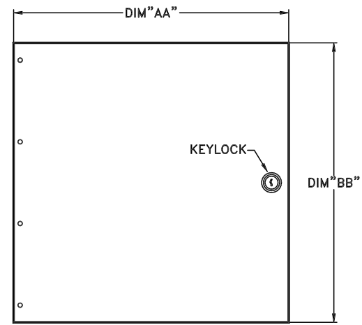
PANEL DOOR .125" ALUMINUM
