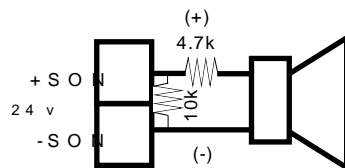
SC616CP Sonalert
